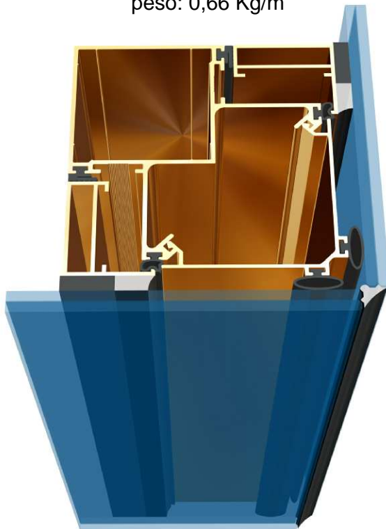
Modelo en 3D - Columna 90° Frente Vidriado Columna 370 y Tapa 371
