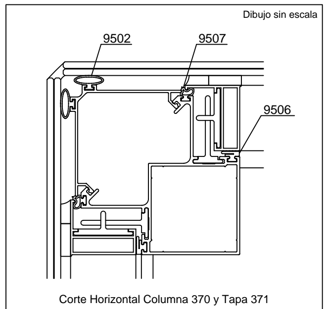
Nuevos perfiles Línea Frente Vidriado, Columna y tapa para esquina 90°
