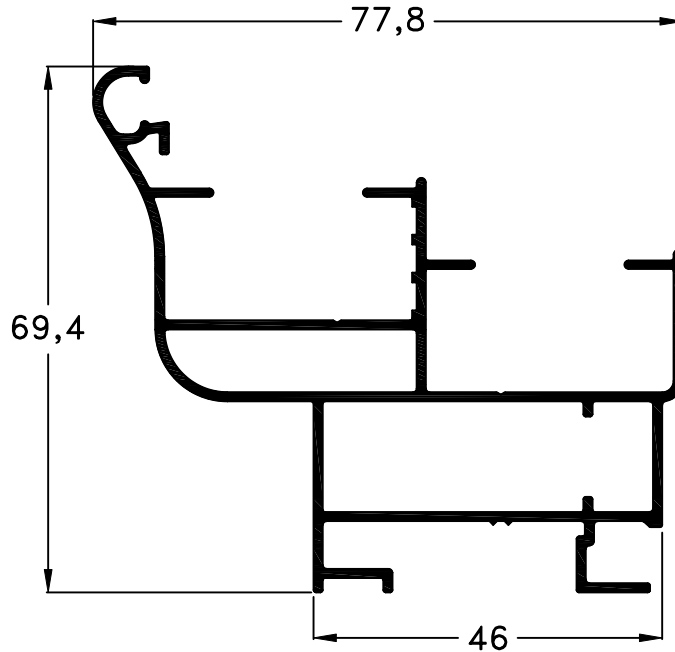
898 - Marco de Ventana Guillotina Largo std.: 6150 mm Peso: 1200 g/m
