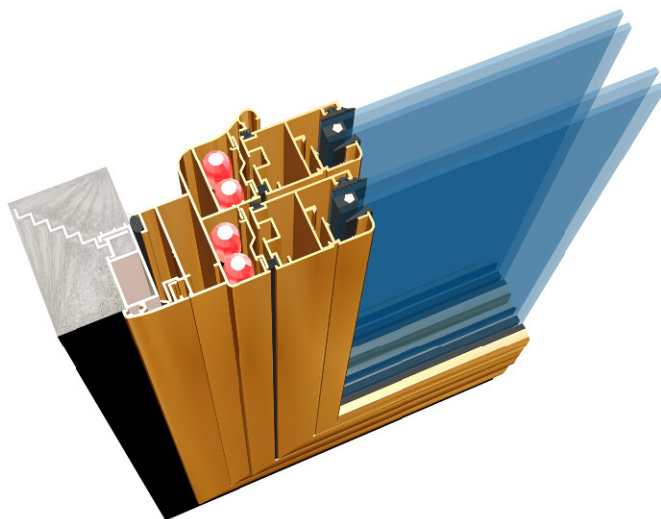
Línea Gamma Marco 505
