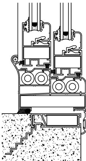
Línea Gamma Marco 505
