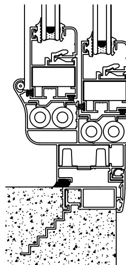
Línea Mónaco Top Marco 898
