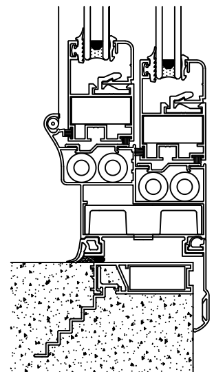
Línea Mediterránea Marco 512
