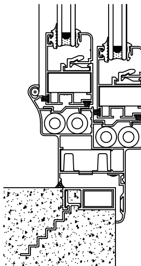
Línea Delta Marco 511
