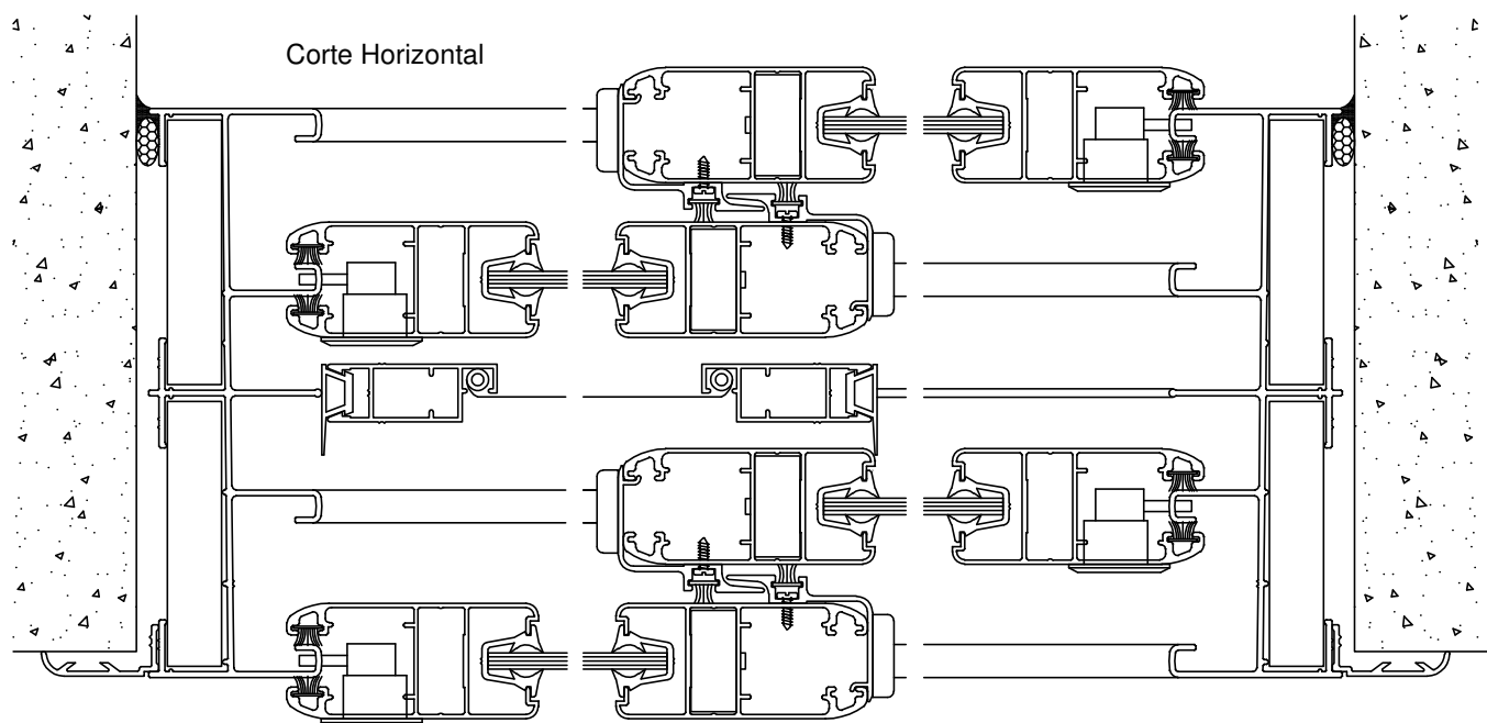
960 - Marco Cuatro Guías peso: 1590 g/m
