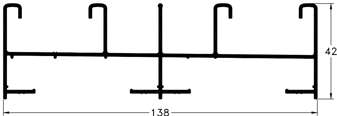
960 - Marco Cuatro Guías peso: 1590 g/m
