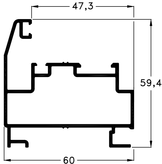
894 - Marco Coplanar M-Tres Peso: 1030 g/m.
