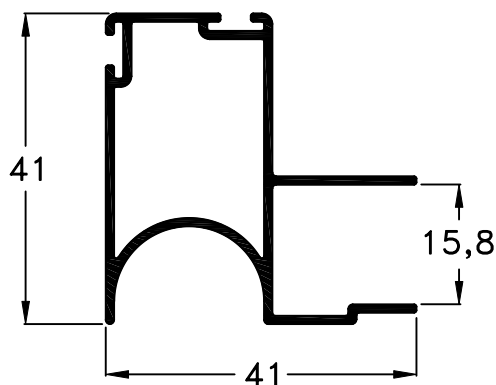
155 - Parante p/15 mm. Largo Std.: 5200 mm. Peso: 550 g/m.
