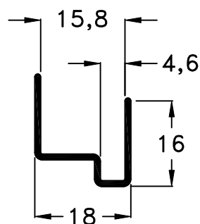
156 - Cantonera p/15 mm. peso: 160 g/m.
