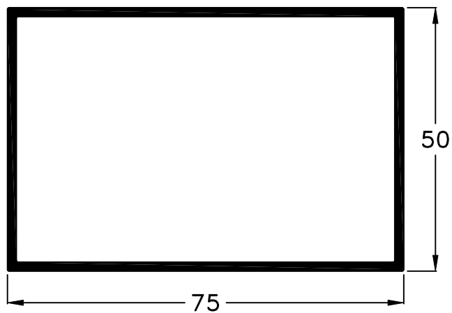
464 - Tubo Rectangular de 75 x 50 mm. Peso: 1120 g/m
