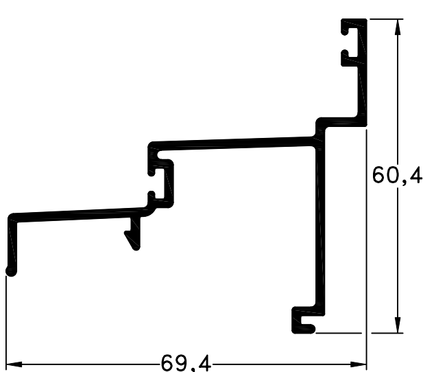
378 - Bota Agua paño Fijo peso: 0,79 Kg/m
