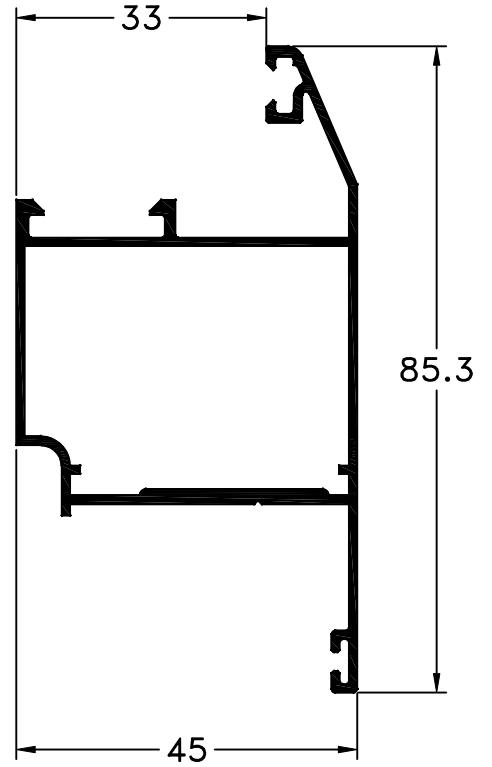
737 - Hoja de Ventana Desplazable peso: 810 g/m
