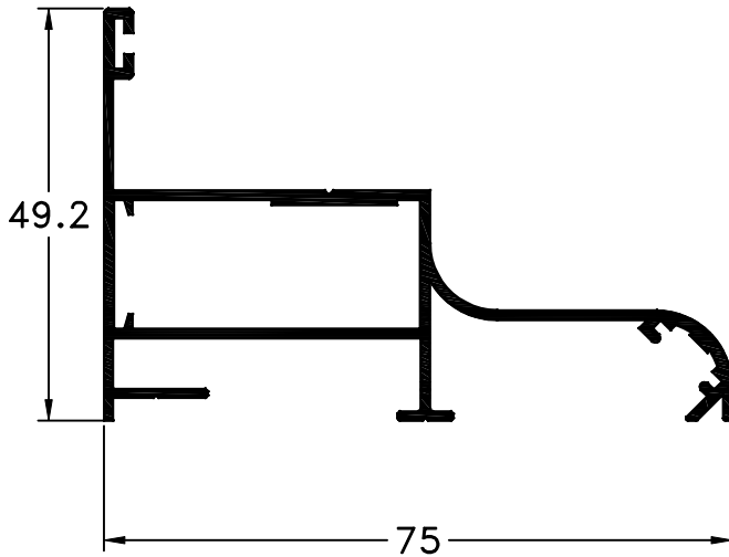
739 - Marco de Ventana Desplazable peso: 770 g/m
