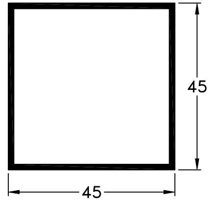
808 - Tubo 45 x 45 mm peso: 0,71 Kg/m
