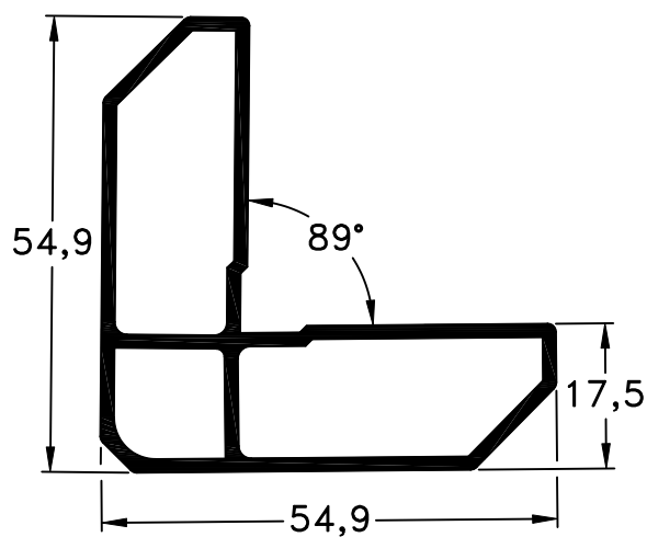
86 - Escuadra Suplementaria peso: 1,00 Kg/m
