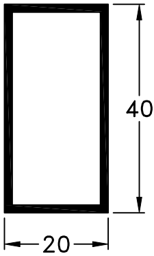
805 - Tubo 40 x 20 mm peso: 0,46 Kg/m
