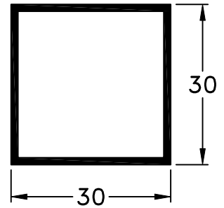
806 - Tubo 30 x 30 mm peso: 0,40 Kg/m
