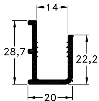
31 - Porta Blisan Inferior Peso: 0,38 Kg/m
