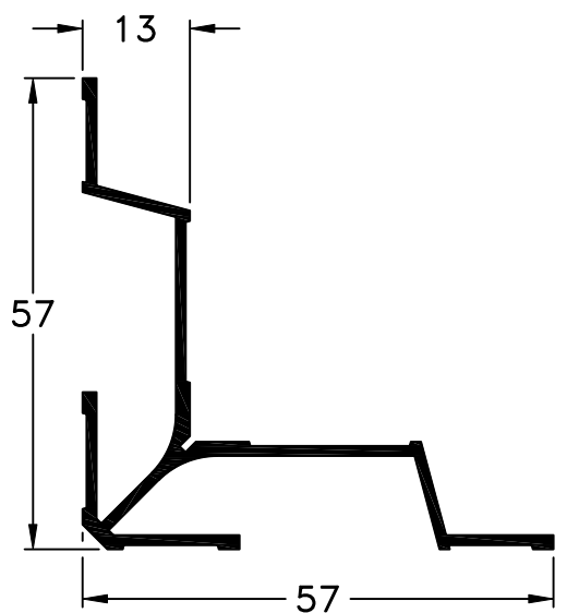
55 - Escuadra Universal Intermedia peso: 0,56 Kg/m
