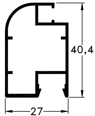
109 - Mosquitero peso: 0,44 Kg/m
