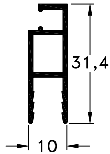
60 - Mosquitero peso: 0,25 Kg/m
