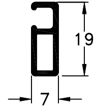
61 - Mosquitero peso: 0,17 Kg/m
