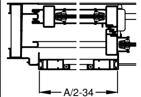
Corte Horizontal A-A
