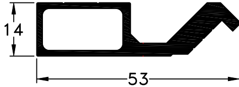
5038 - Bisagra (Alcemar) peso: 0,72Kg/m
