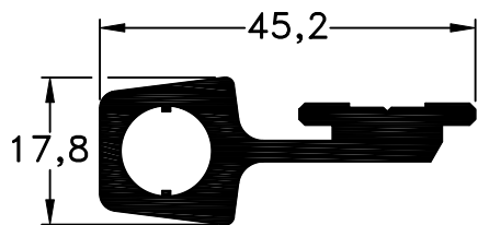
5414 - Bisagra H33 cuadrada peso: 0,81Kg/m
