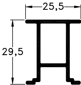
5575 - Cuna Multipunto M5 peso: 0,42Kg/m
