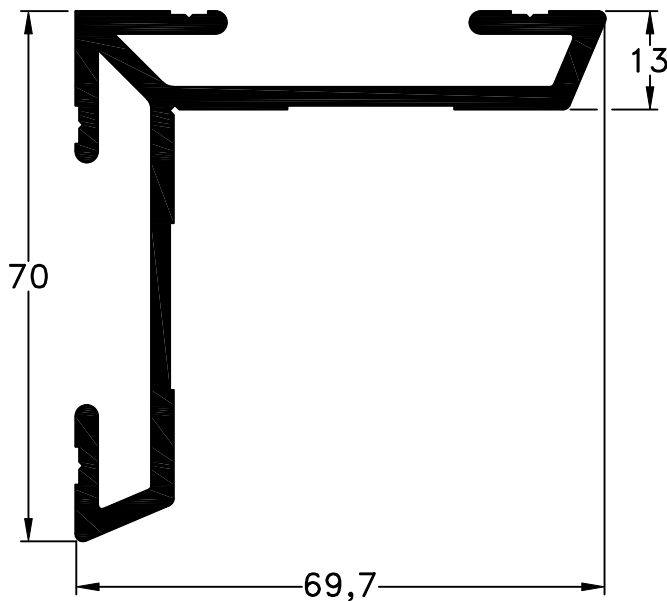
5045 - Escuadra Pesada peso: 1,56Kg/m
