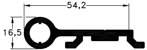
5434 - Bisagra BTA peso: 0,95Kg/m
