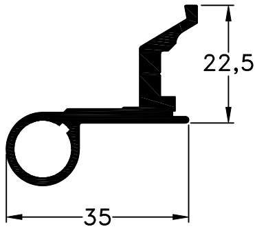
5036 - Bisagra (Panizza) peso: 0,60Kg/m
