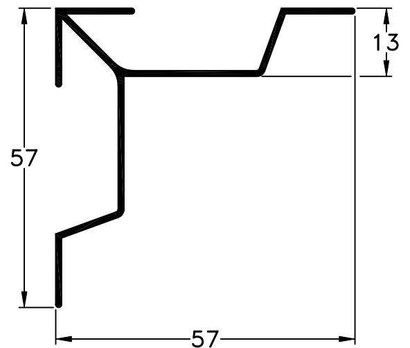
5046 - Escuadra Universal peso: 0,45Kg/m
