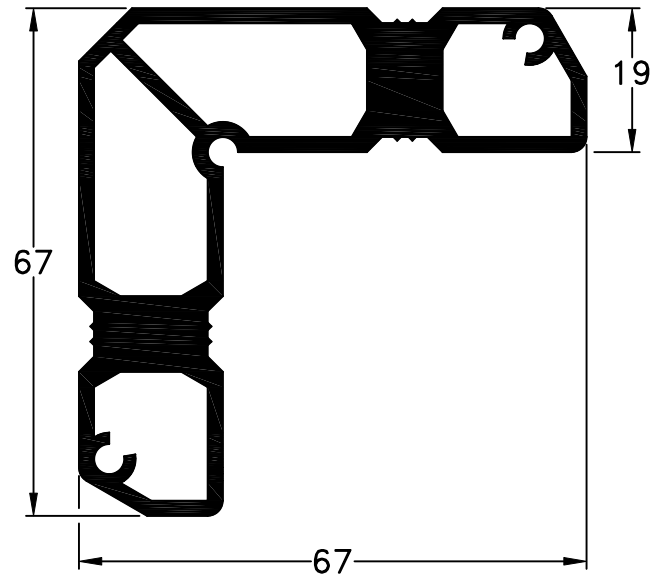
5068 - Escuadra Extruida de Expansión de 19 peso: 2,22Kg/m
