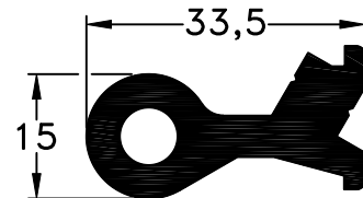
5435 - Perfil Para Accesorio E-71 peso: 0,83Kg/m
