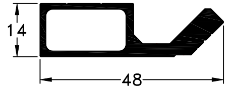
5039 - Bisagra (Alcemar) peso: 0,64Kg/m
