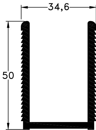
5445 - U de Armado 90x40 peso: 1,10Kg/m
