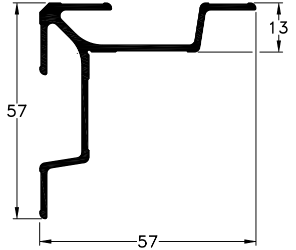
5063 - Escuadra peso: 0,74Kg/m
