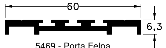
5469 - Porta Felpa peso: 0,55Kg/m
