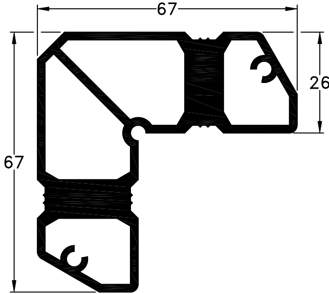
5069 - Escuadra Extruida de Expansión de 26 peso: 2,63Kg/m
