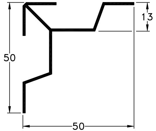
5040 - Escuadra Universal peso: 0,40Kg/m
