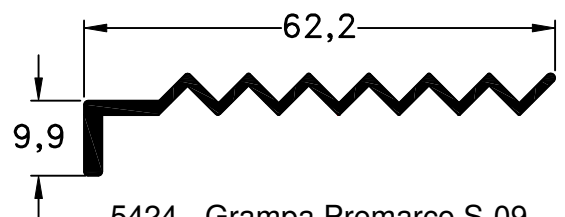
5424 - Grampa Premarco S-09 peso: 0,42Kg/m
