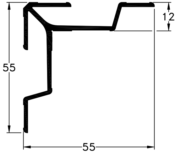
5062 - Escuadra Premarco peso: 0,68Kg/m
