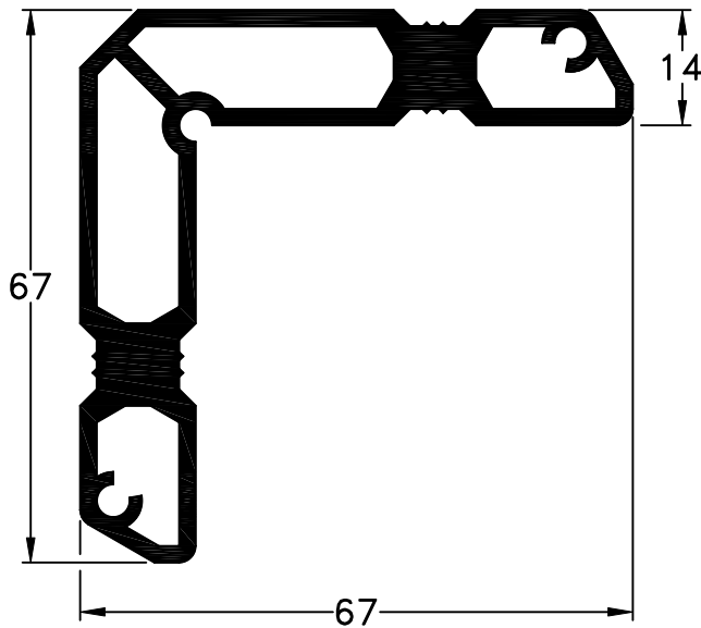
5067 - Escuadra Extruida de Expansión de 14 peso: 1,92Kg/m
