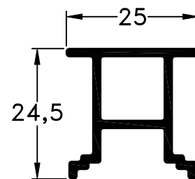
5576 - Cuna Multipunto M3 peso: 0,37Kg/m
